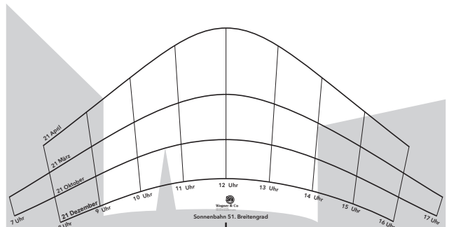
Bild 5 Die Gebäude und Baumumrisse können Sie auf die Sonnenbahnfolie oder auf eine zweite dahintergeklebte Folie mittels wasserlöslichem Folienschreibers aufzeichnen. Den zukünftigen Standort der Solaranlage aufsuchen.
